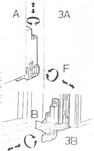
Valsluitplaat
